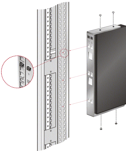
Abbildung 2-1. Installation der 0-HE-Befestigungshalterung
