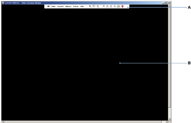
Abbildung 4-2. Viewer-Fenster
